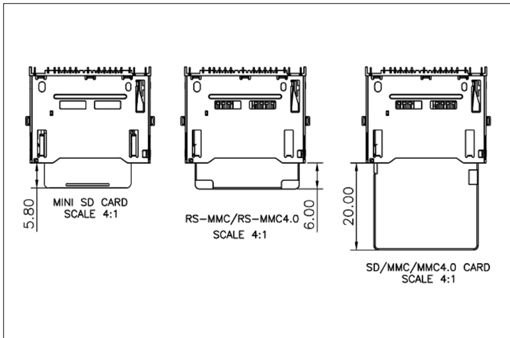
CS-601 (六合一卡座)
